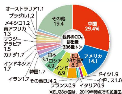
▲図2 世界のエネルギー起源 CO 2 排出量の国別内訳 (2019年。環境省資料による)
