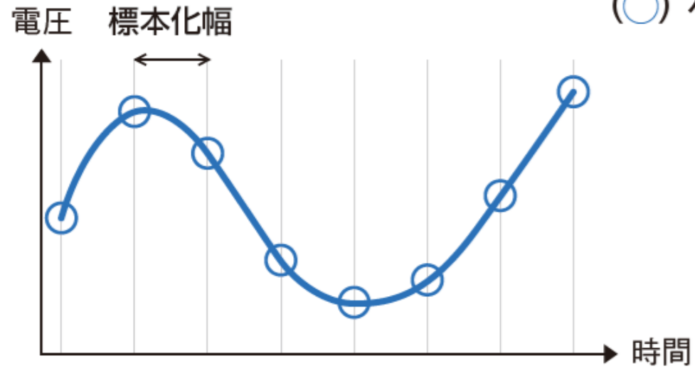
(1) 標本化 (サンプリング)
